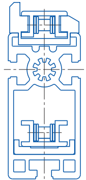
BS60 Scharnierbandkette*/ Hinge chain*/ Convoyeur à chaînes charnières*
